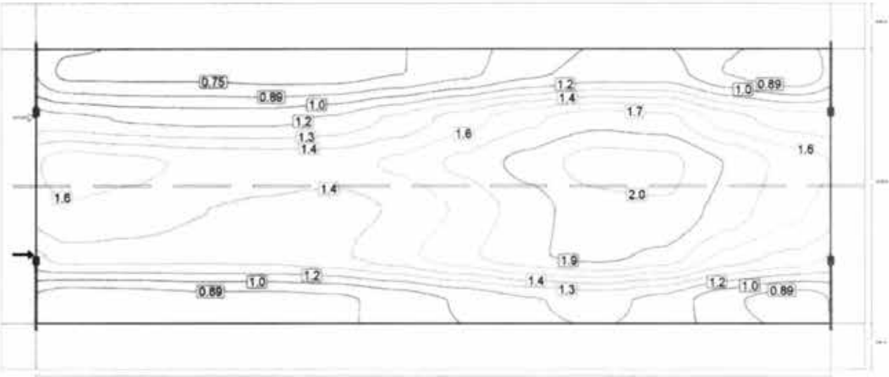
Observador 1: Valor de manutenção de luminância com via de rodagem seca [cd/m²] (Linhas de isolux)
