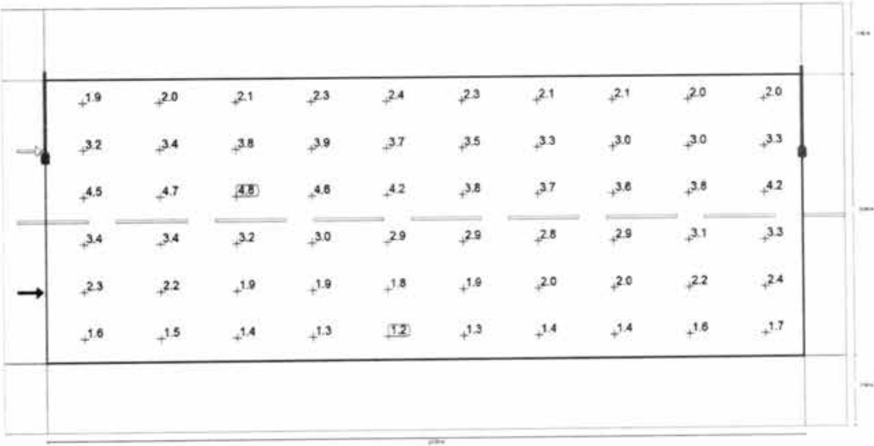
Observador 1: Luminância com instalação nova [cd/m²] (Grelha de valores)
