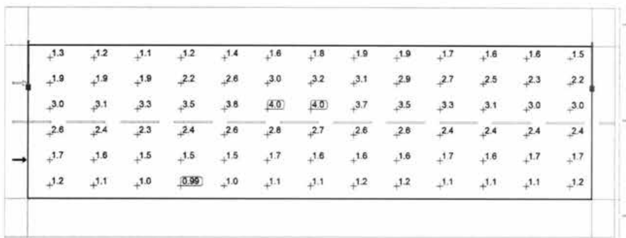
Observador 1: Luminância com instalação nova [ \text{cd}/\text{m}^2 ] (Grelha de valores)
