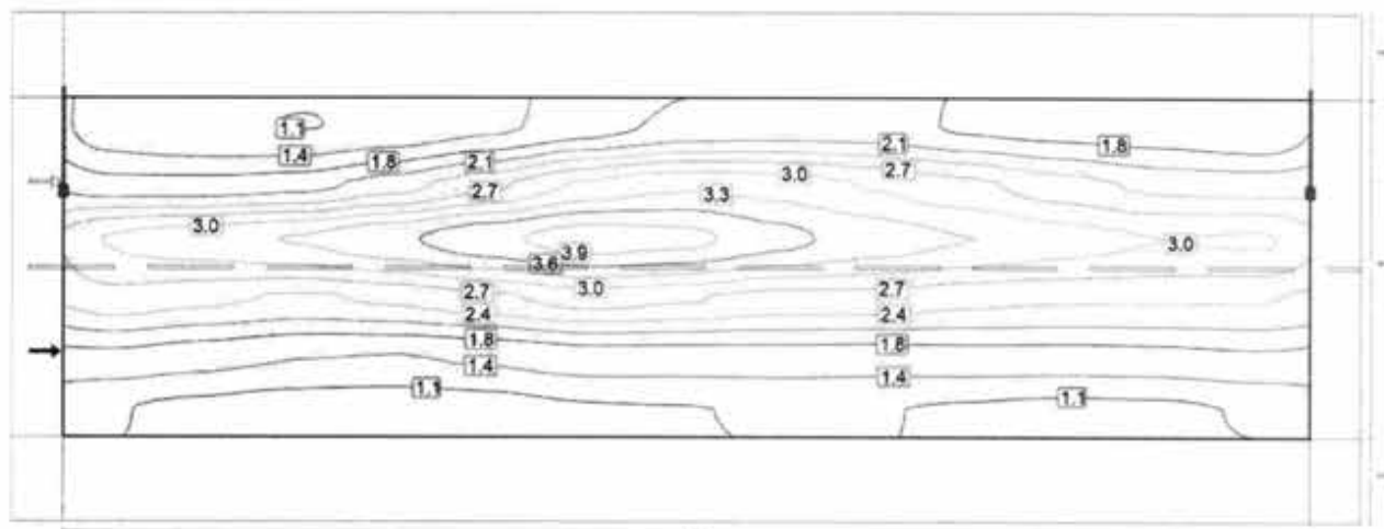
Observador 1: Luminância com instalação nova [ \text{cd}/\text{m}^2 ] (Linhas de isolux)
